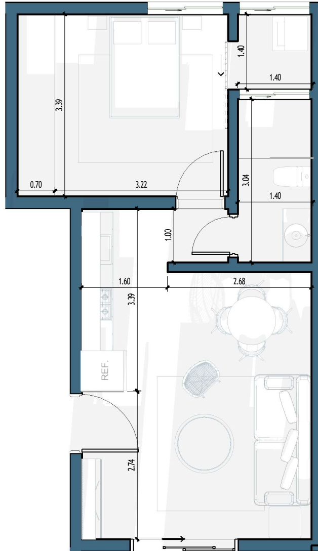
1 C-102 1 : 50
