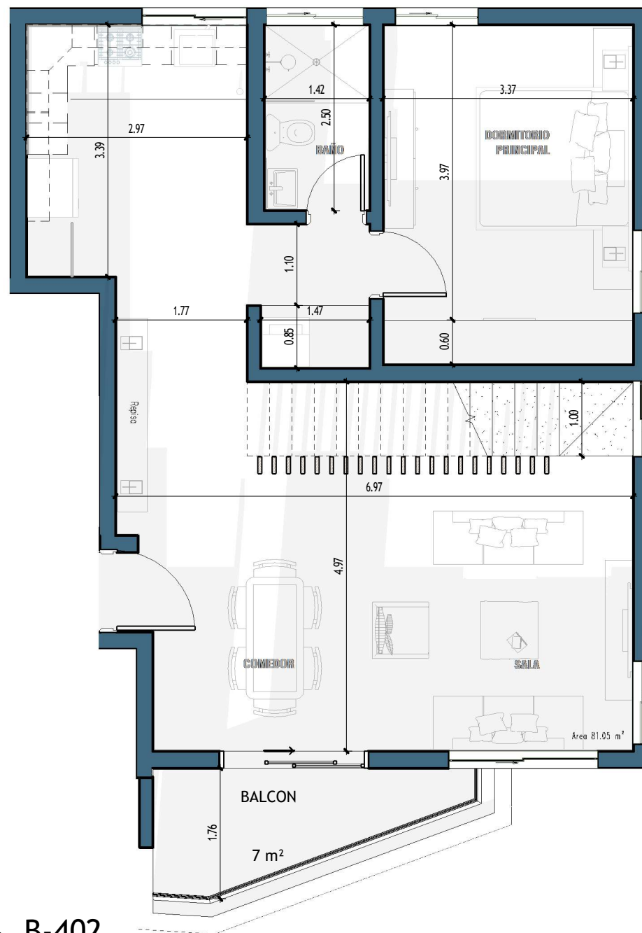
1 B-402 1 : 50
