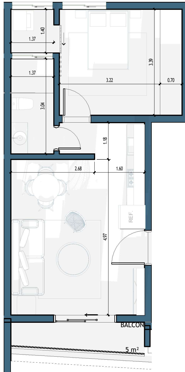
1 D-201 1 : 50
