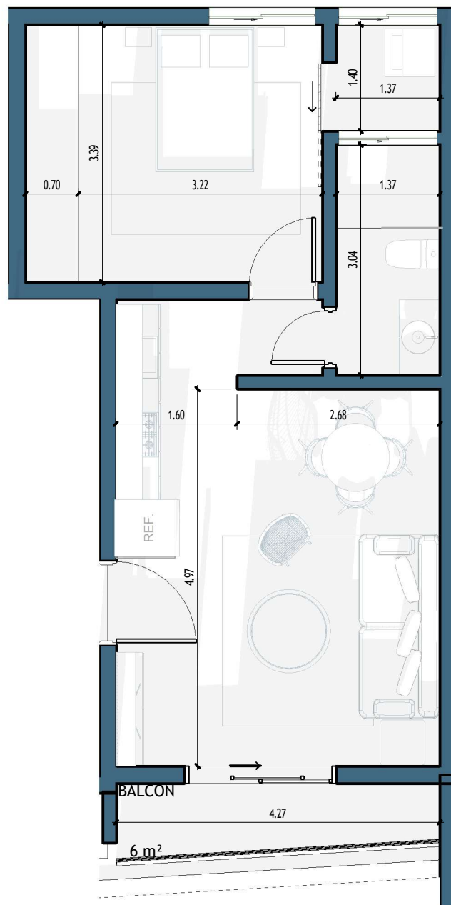
1 A-202 1 : 50
