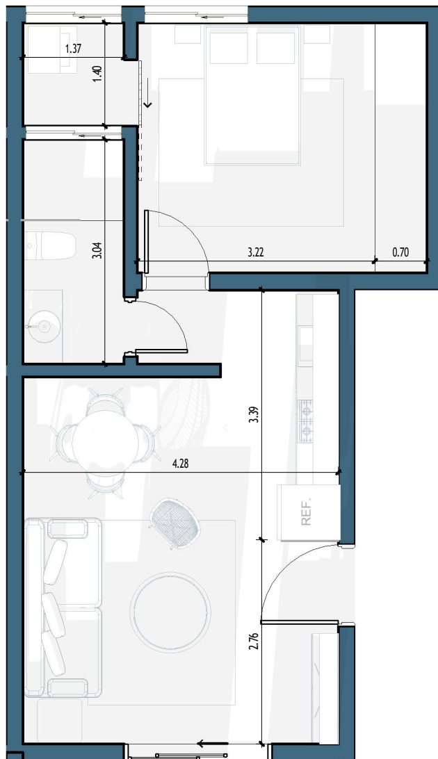
1 D-101 1 : 50
