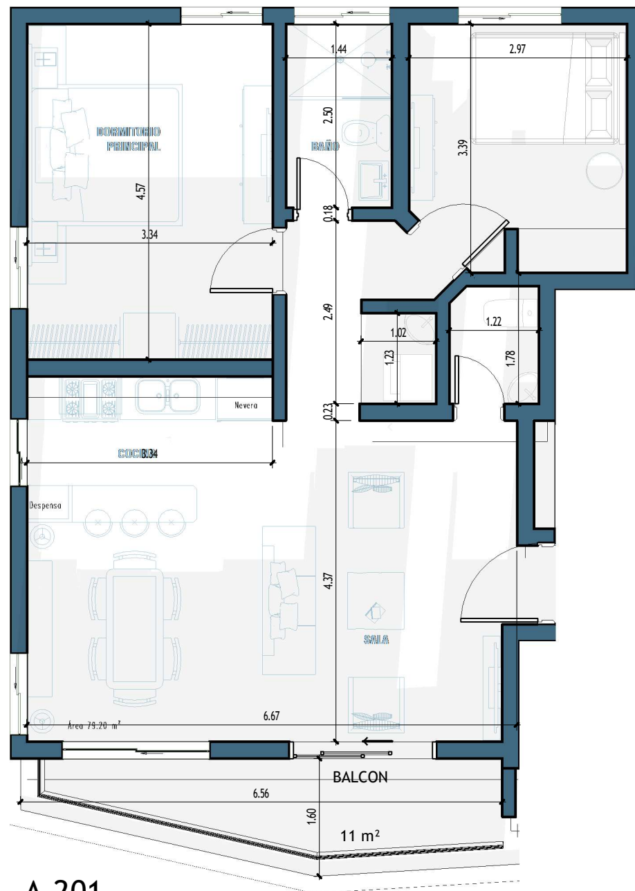
1 A-201 1 : 50
