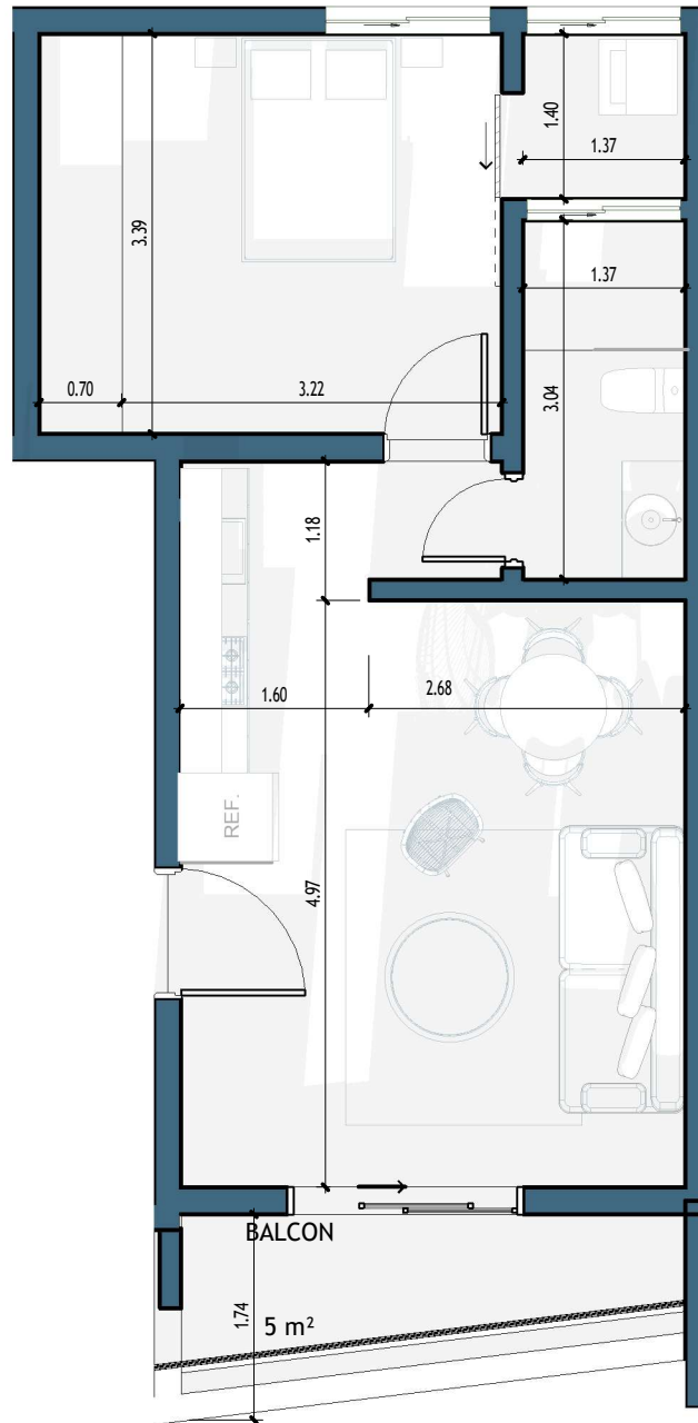
1 C-202 1 : 50
