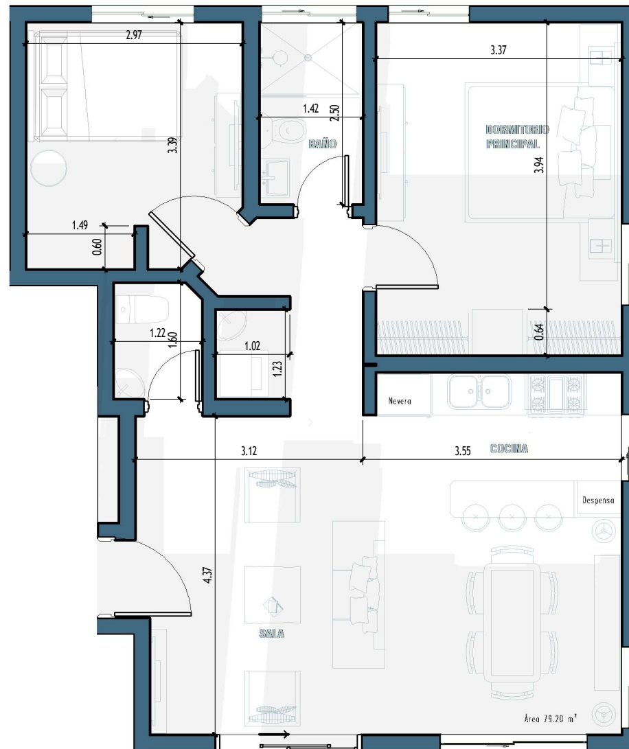
1 B-102 1 : 50
