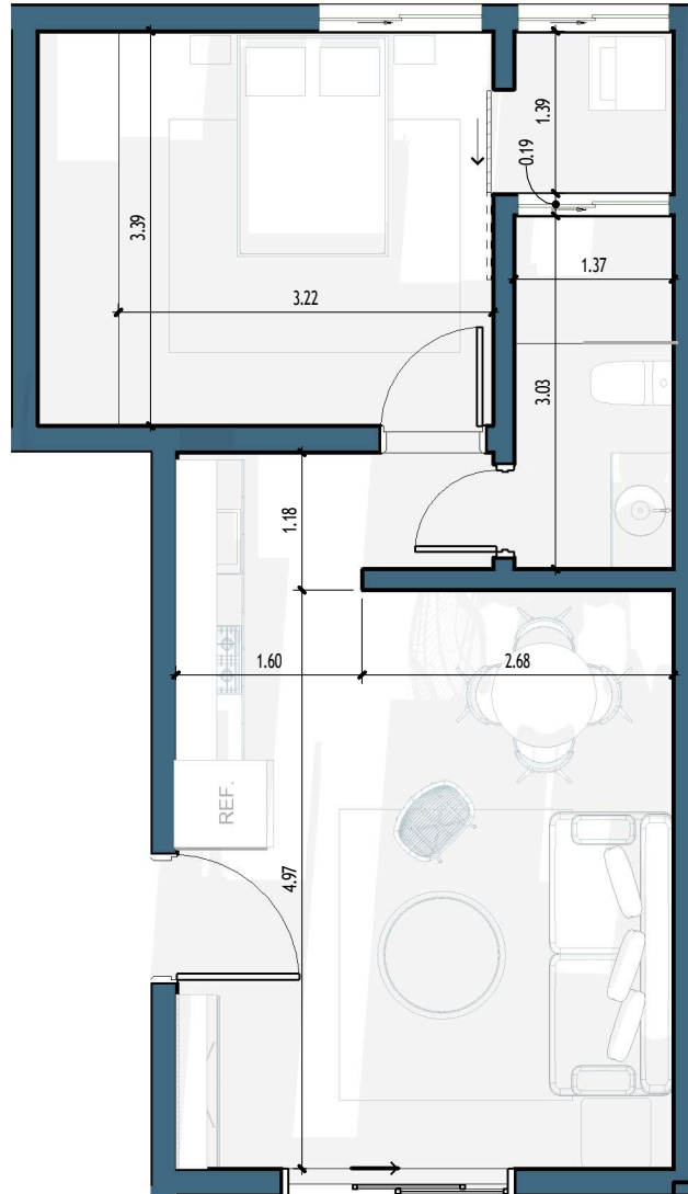
1 A-102 1 : 50
