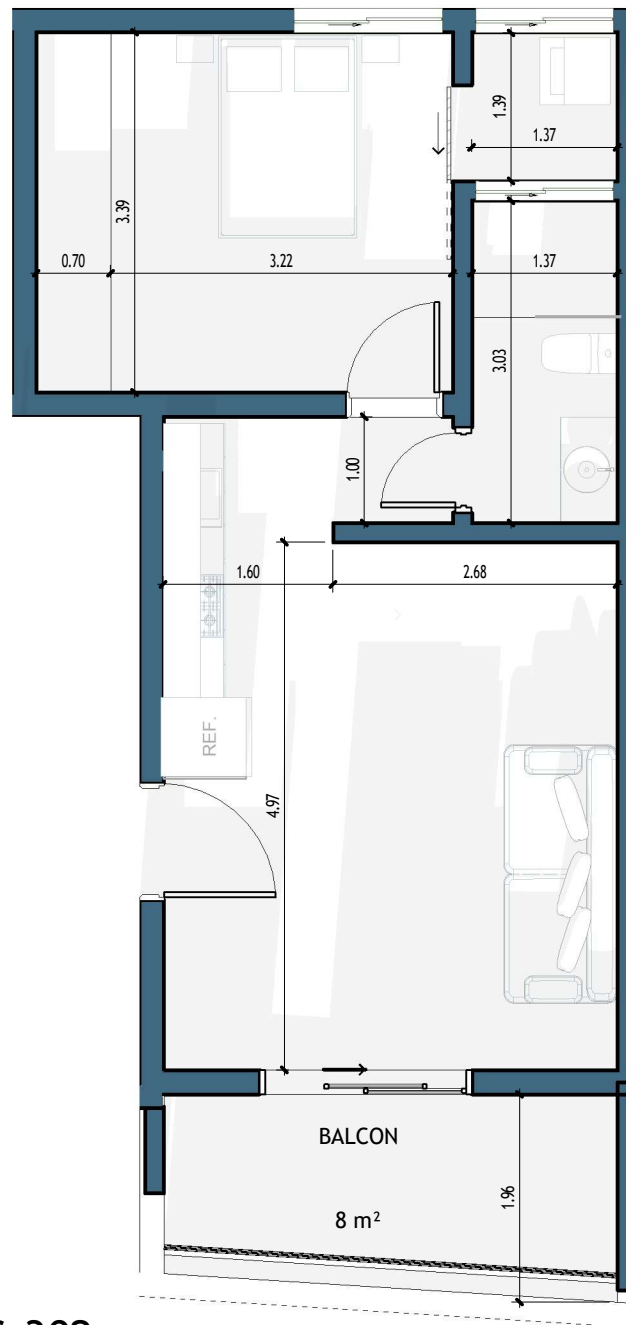
1 C-302 1 : 50
