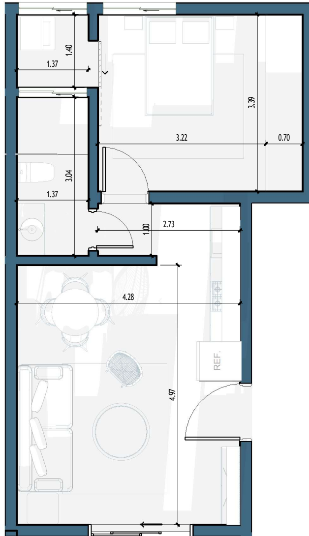
1 B-101 1 : 50
