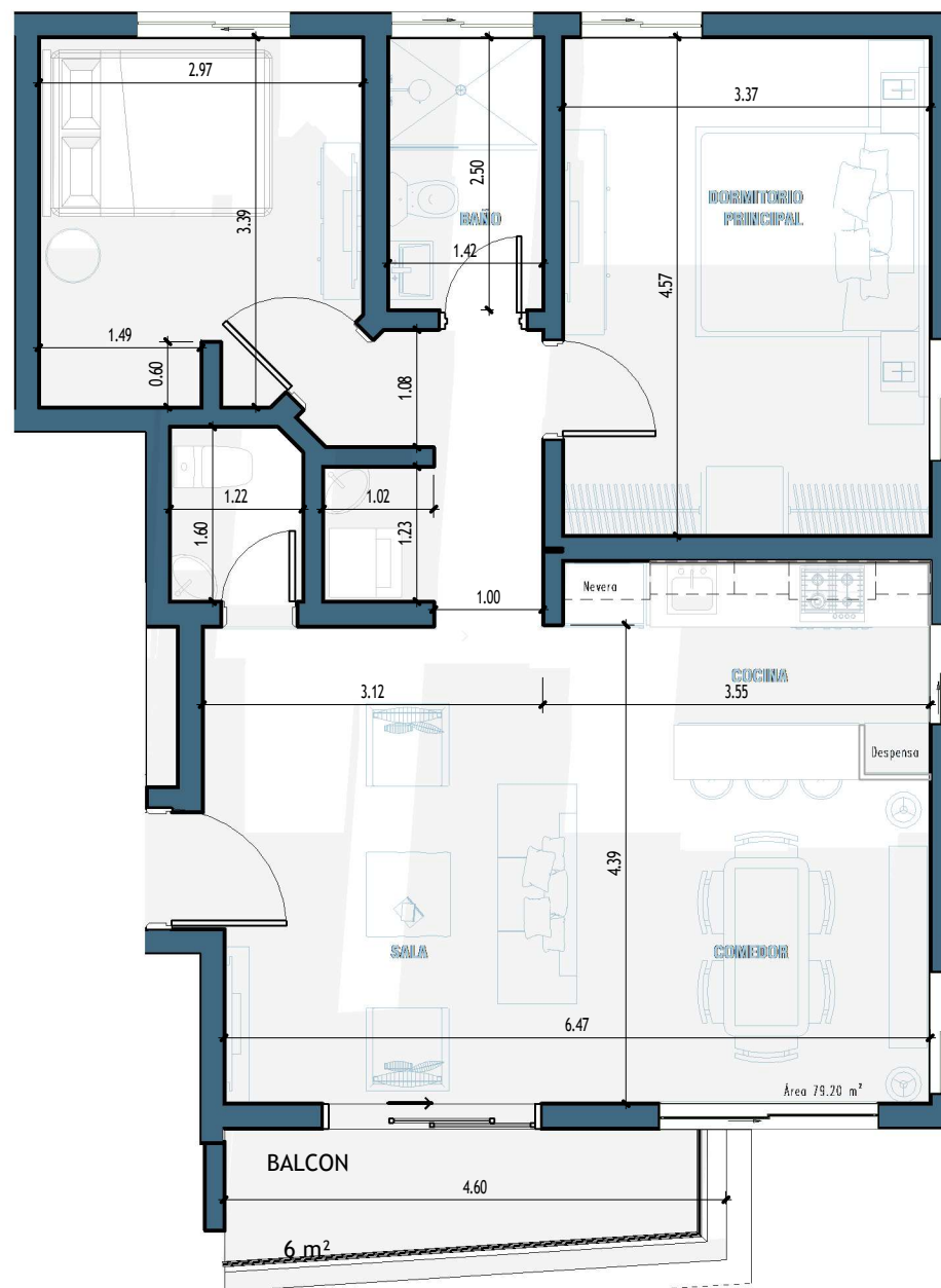
1 B-302 1 : 50
