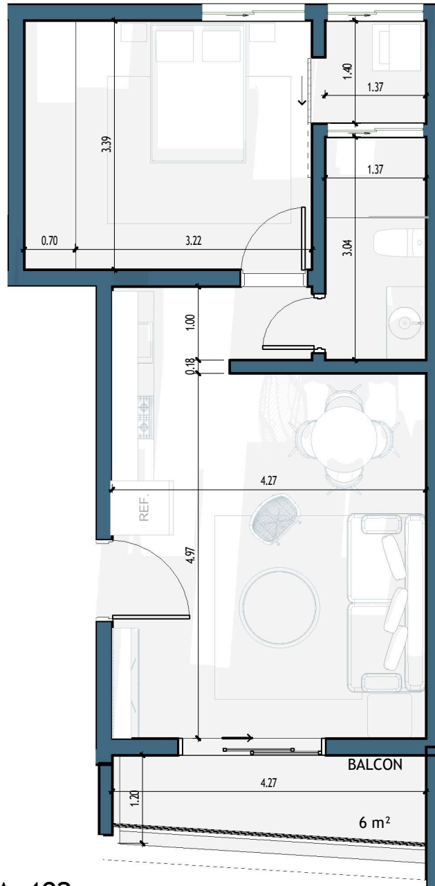
1 A-402 1 : 50
