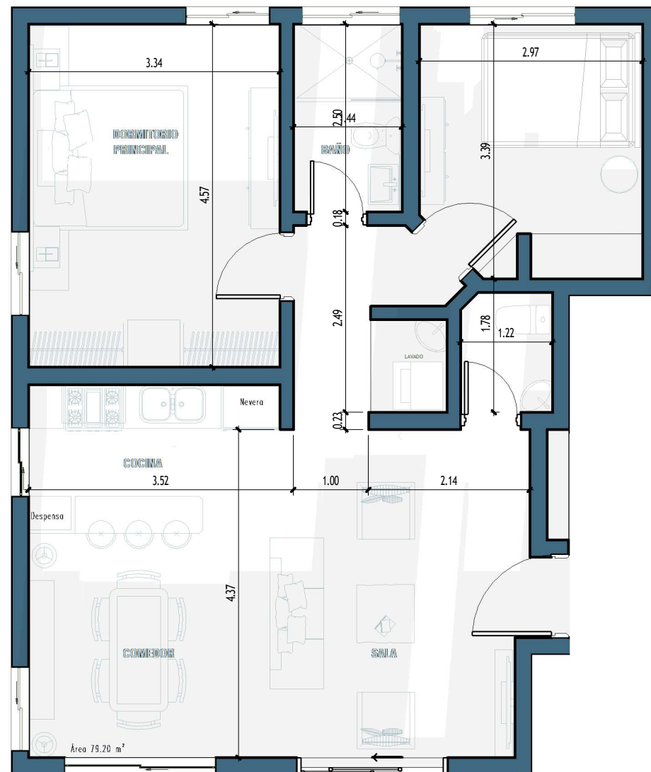
1 A-101 1 : 50
