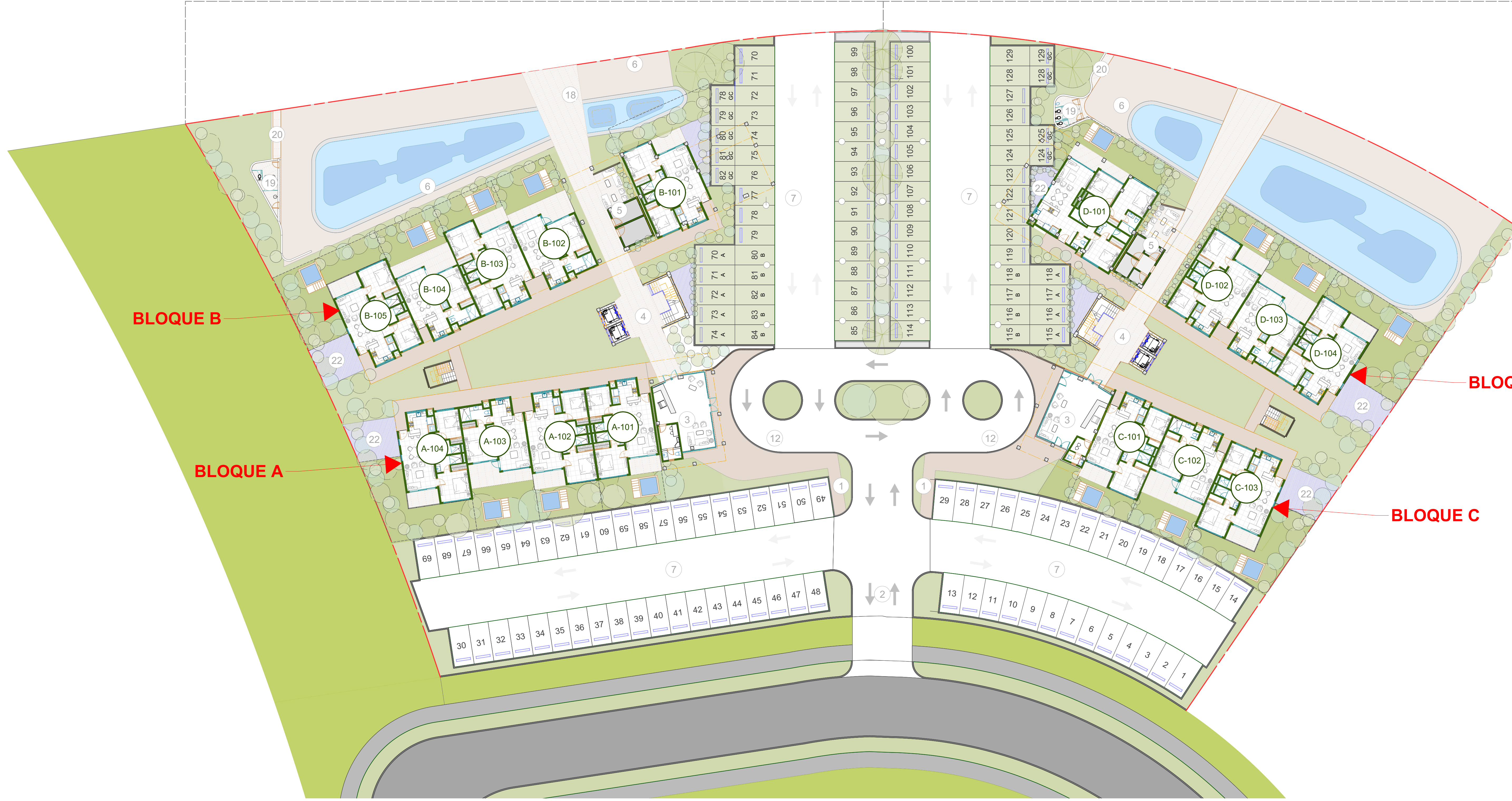
1 PLANTA CONJUNTO - PRIMER NIVEL A141 Scale: 1:250
