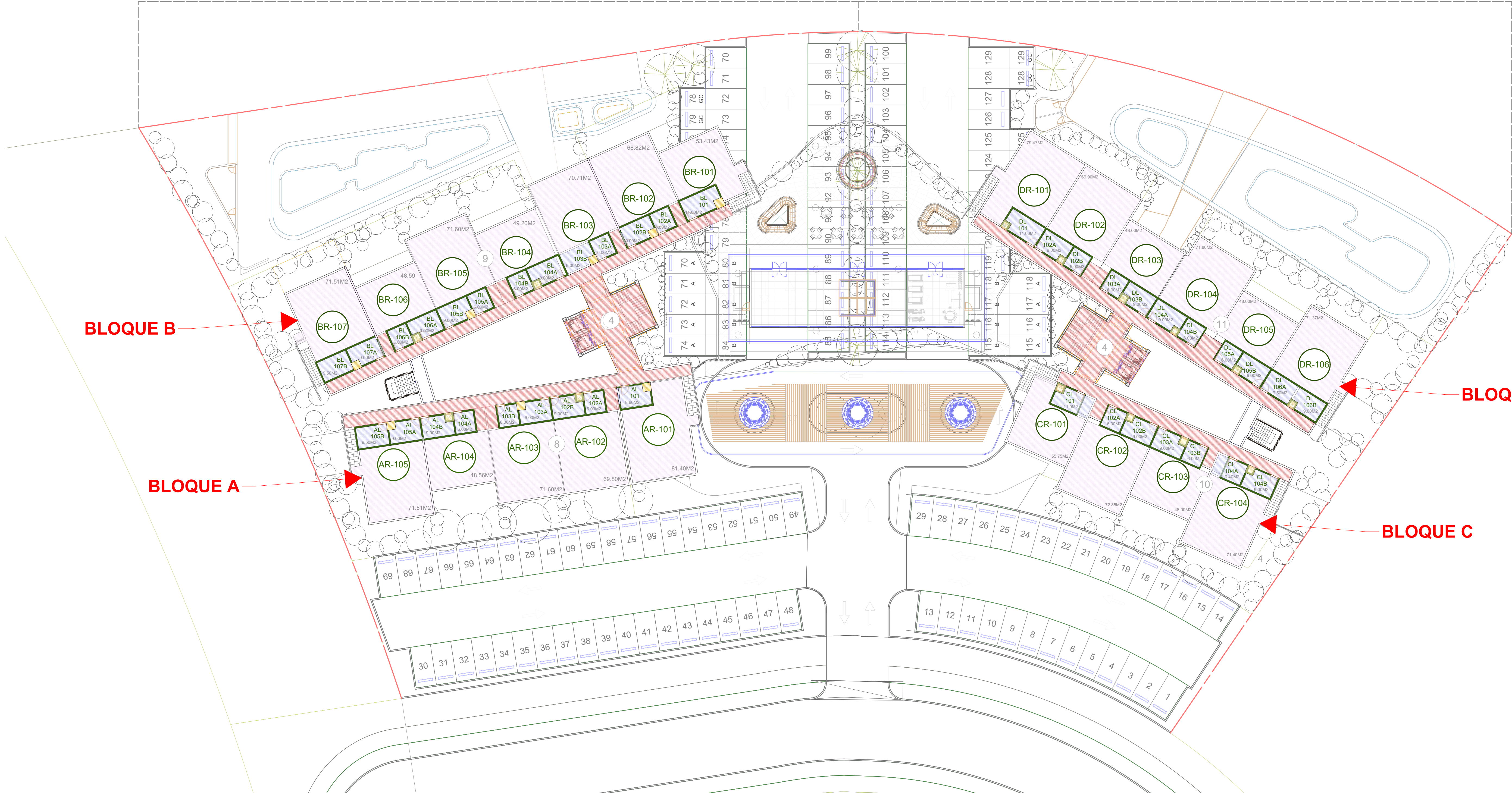
1 PLANTA 5TO NIVEL - BLOQUES APARTAMENTOS A145 Scale: 1:250
