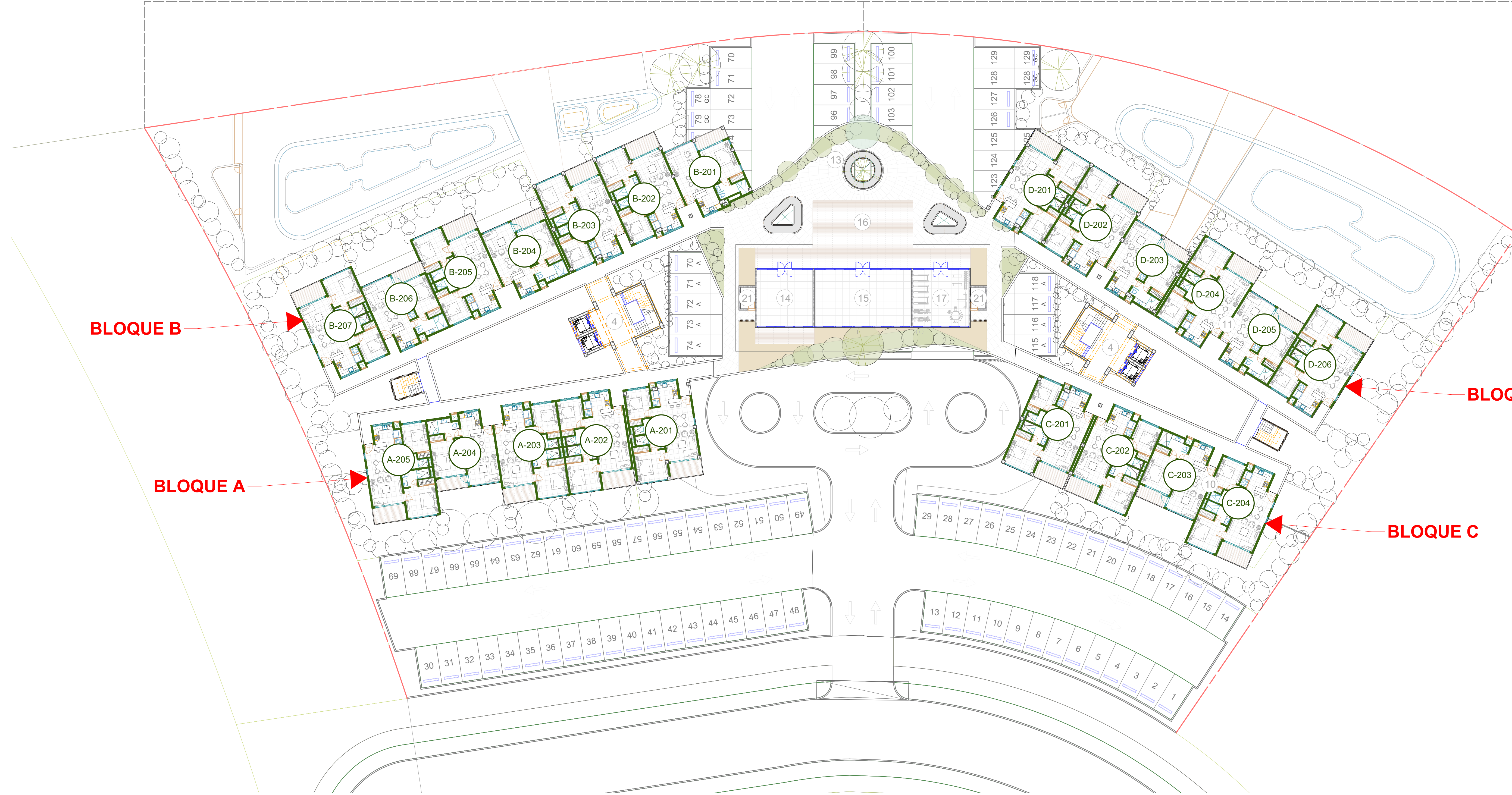
1 PLANTA 2DO NIVEL - ÁREA SOCIAL Y APARTAMENTOS A142 Scale: 1:250
