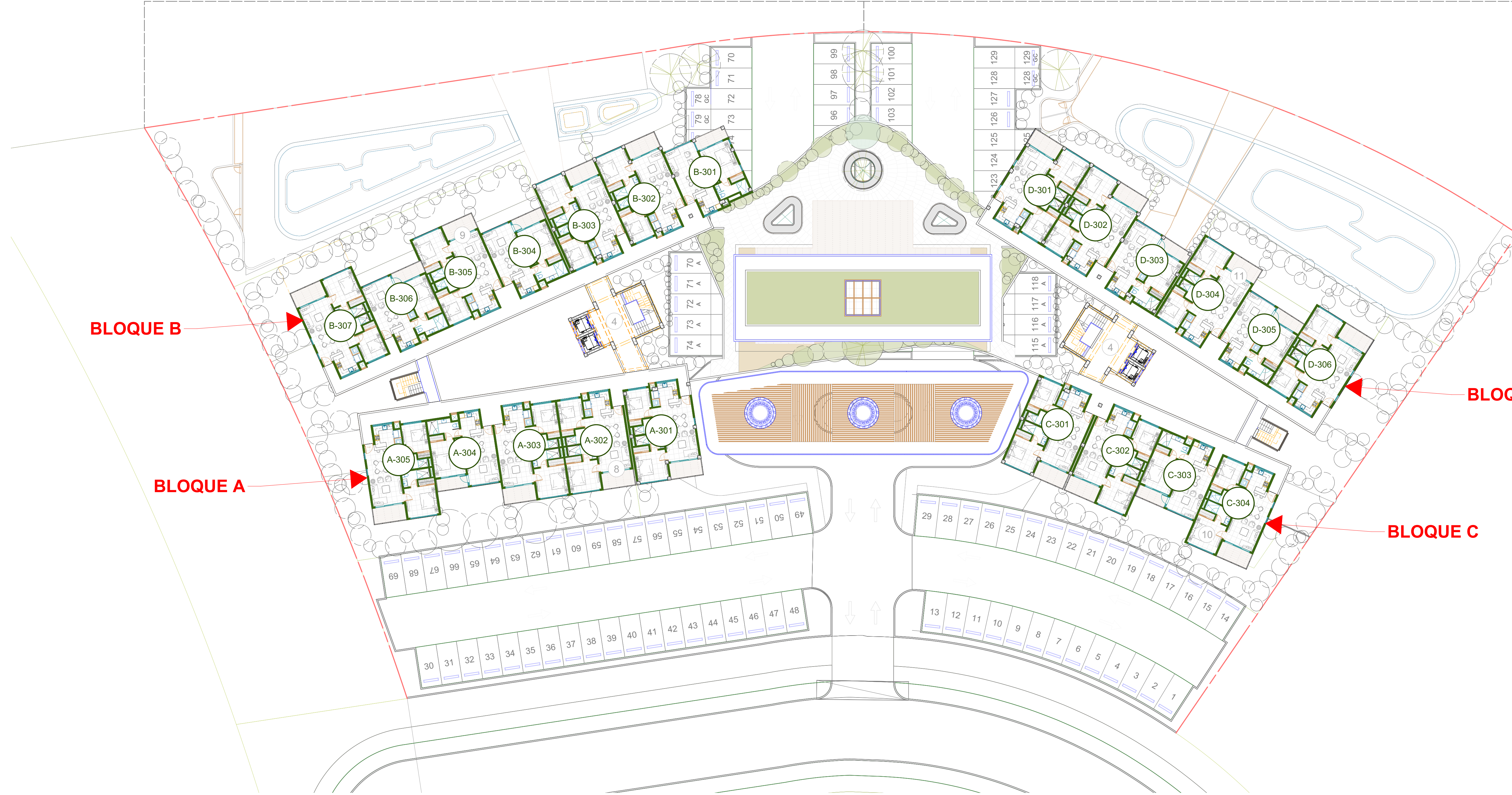
1 PLANTA 3ER NIVEL - BLOQUES APARTAMENTOS A143 Scale: 1:250
